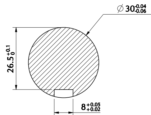
SEZIONE B-B SCALA 1:1
